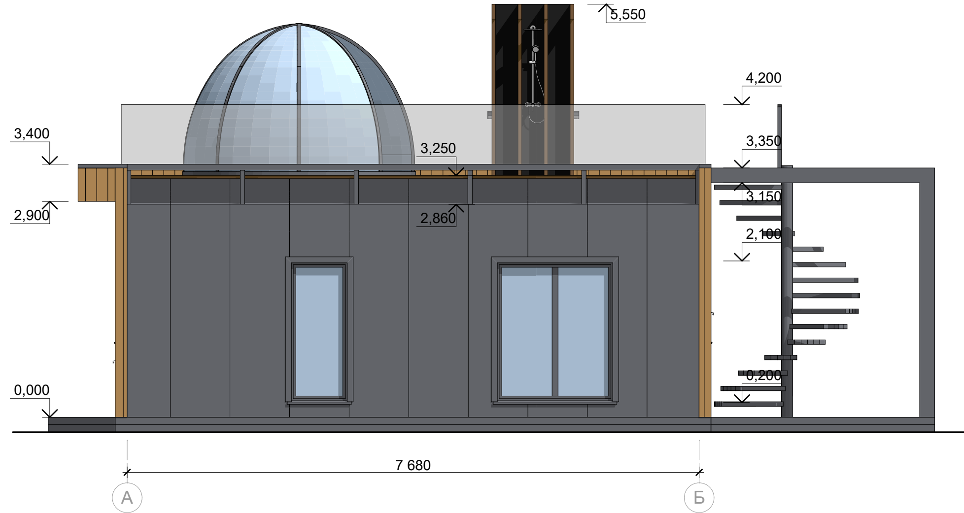
Фасад А-Б
