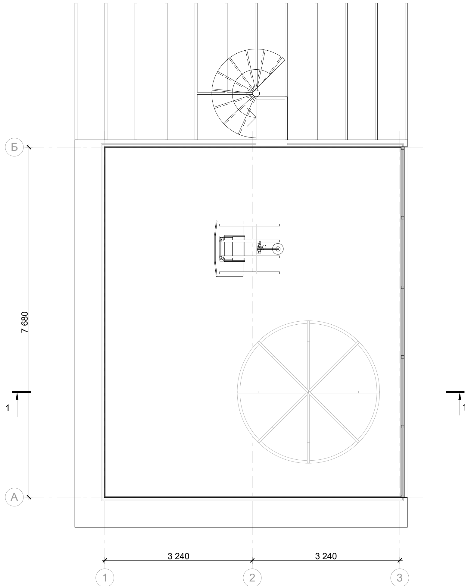
План кровли
