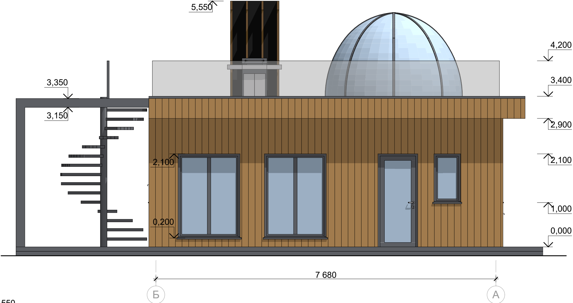
Фасад Б-А
