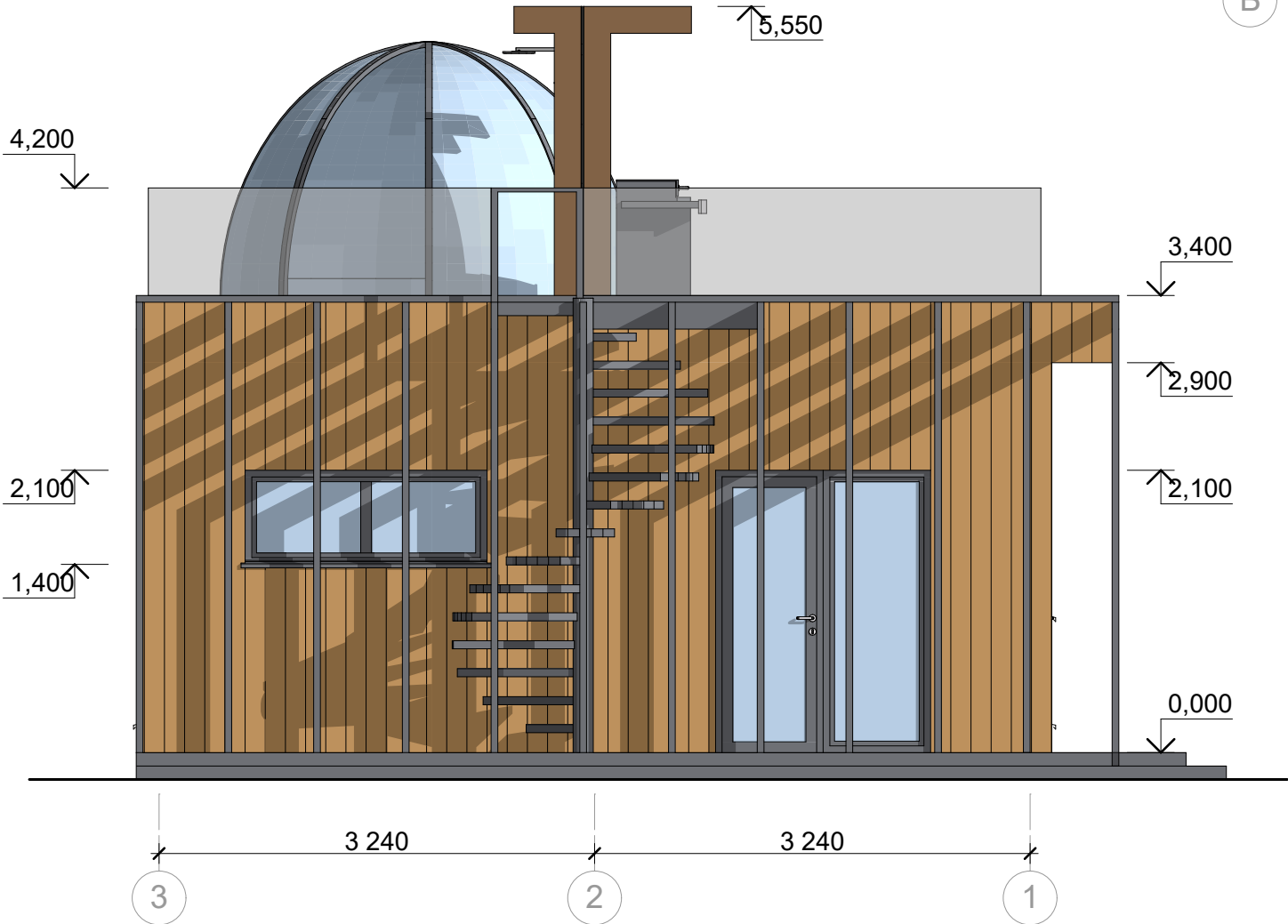
Фасад 3-1
