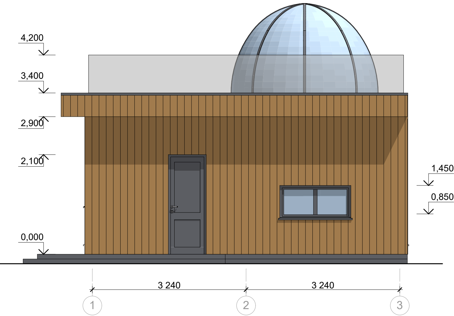
Фасад 1-3
