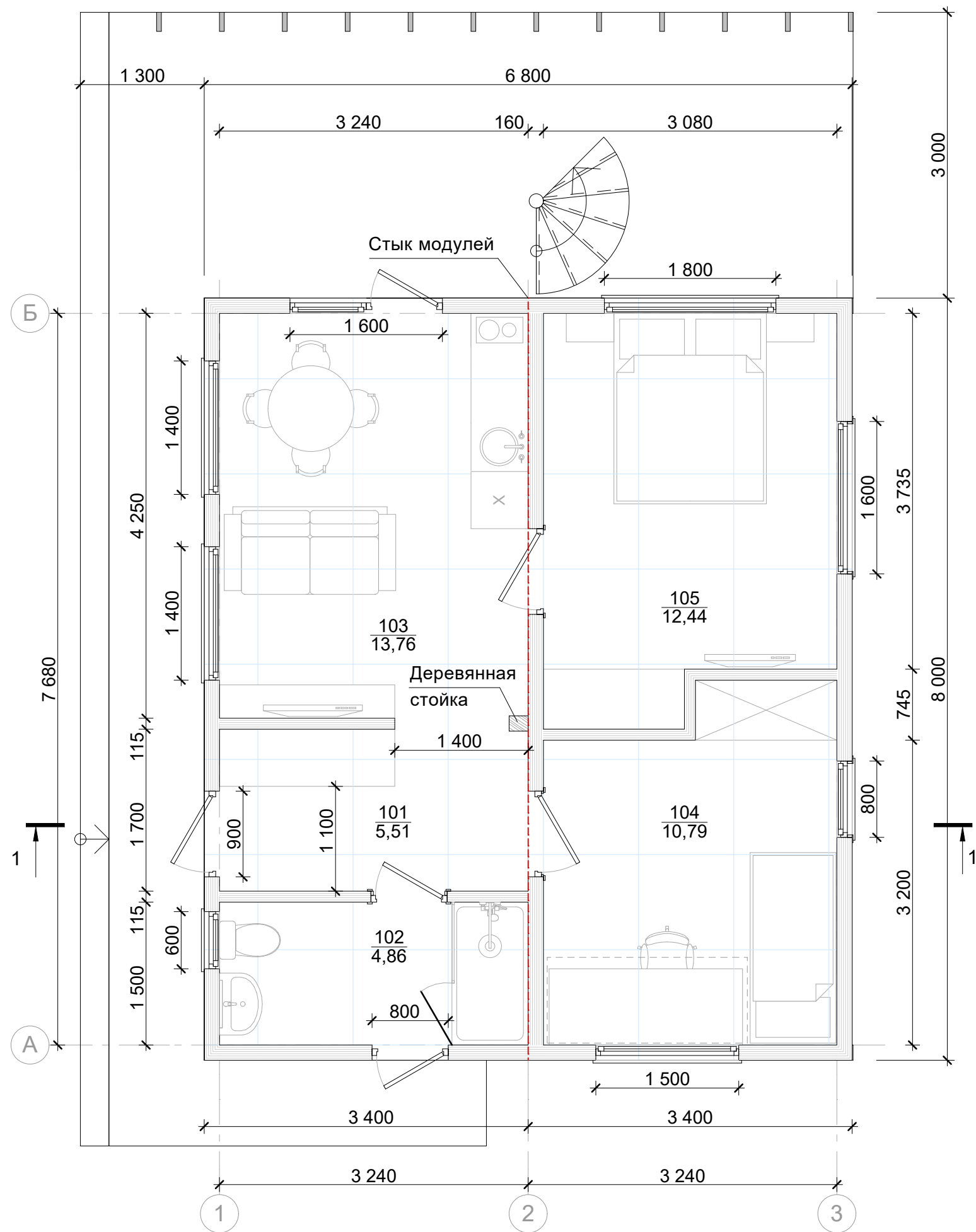
План на отм. 0.00
