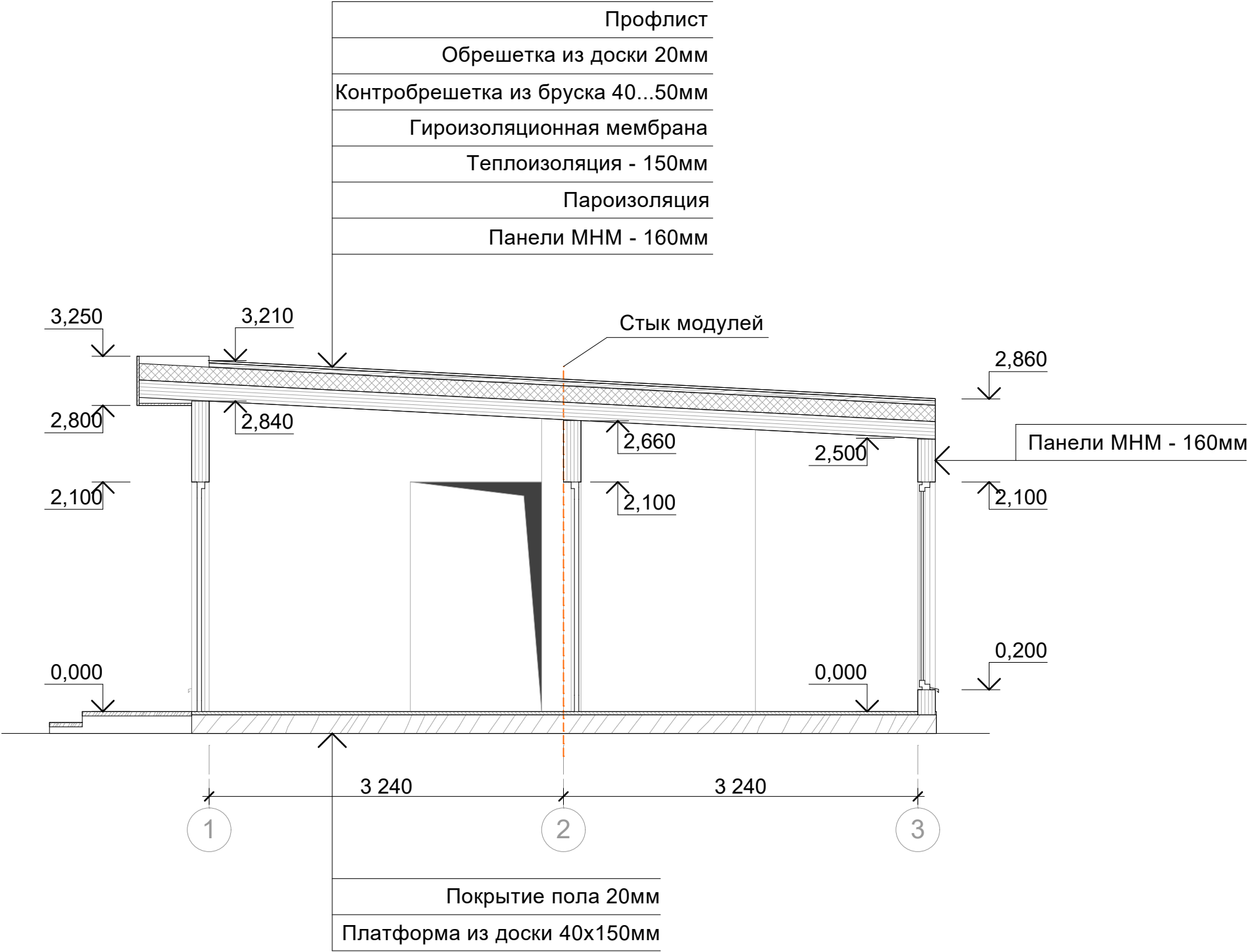
Разрез 1-1
