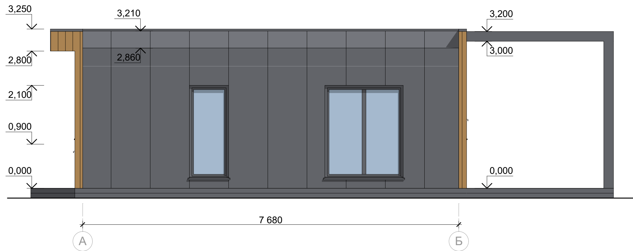
Фасад А-Б
