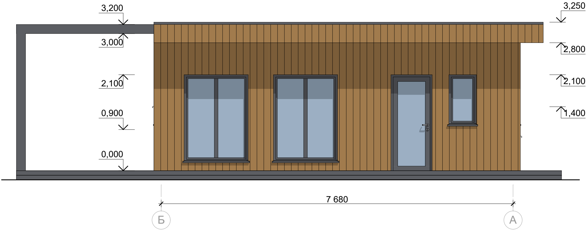
Фасад Б-А
