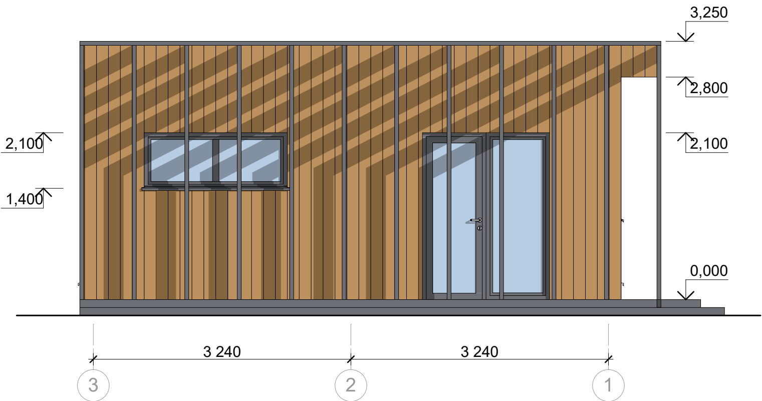
Фасад 3-1
